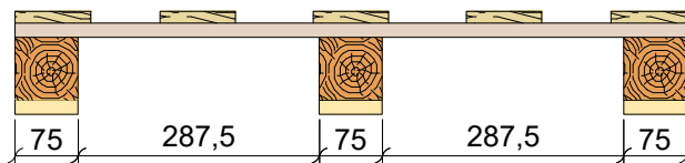
VISTA FRONTALE 1 : 10
