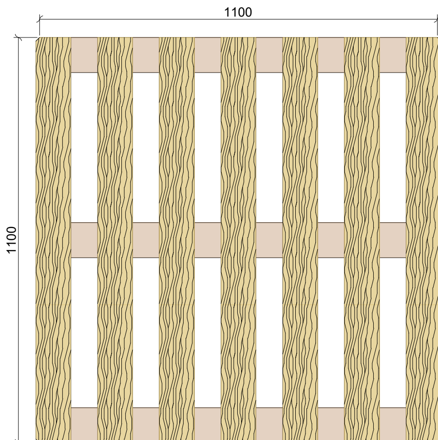
VISTA DA SOPRA 1 : 10
