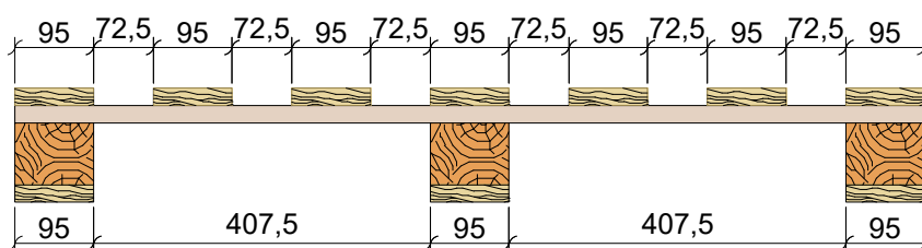
VISTA FRONTALE 1 : 10
